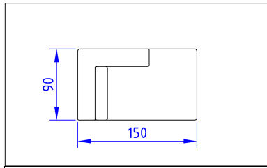
chaise longue A Life P 150 ghost
